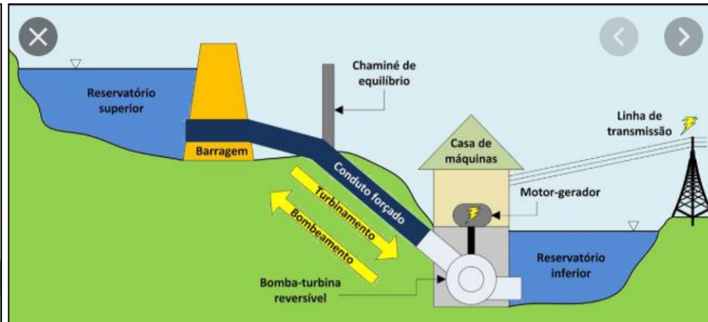
Usina Hidrelétrica Reversível-UHR
