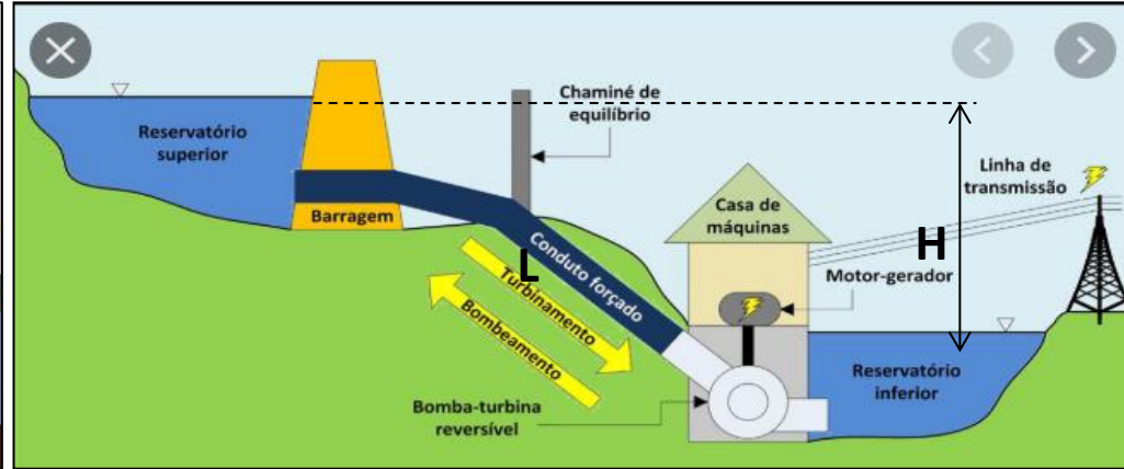
Usina Hidrelétrica Reversível-UHR
