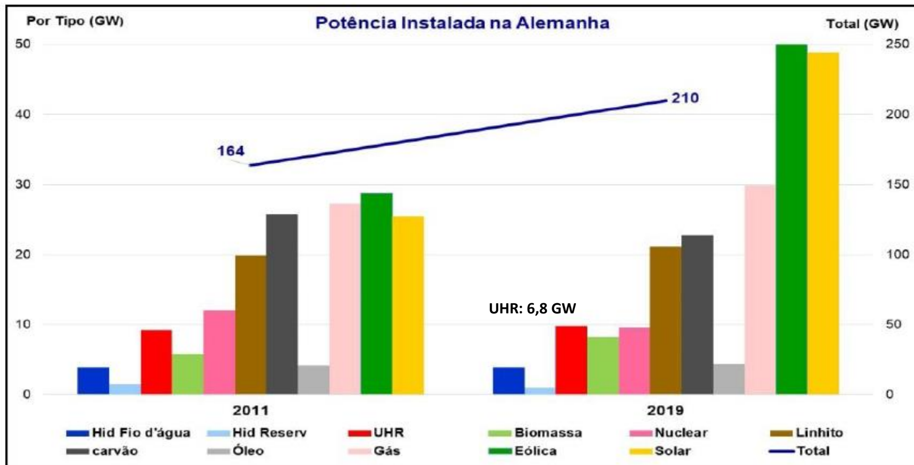
Figura 4.11: Potência Instalada na Alemanha
