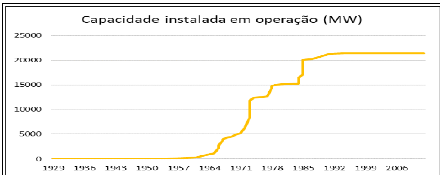
Figura 5.2 - Evolução da capacidade instalada de UHRs nos EUA
