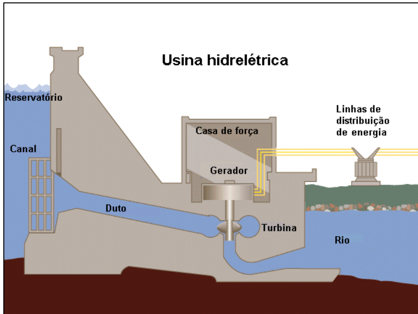
Usina Hidrelétrica Convencional-UHE
