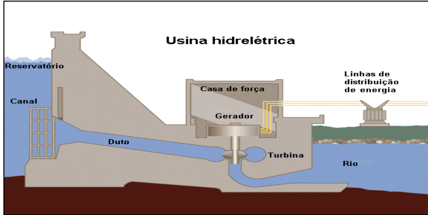
Usina Hidrelétrica Convencional-UHE
